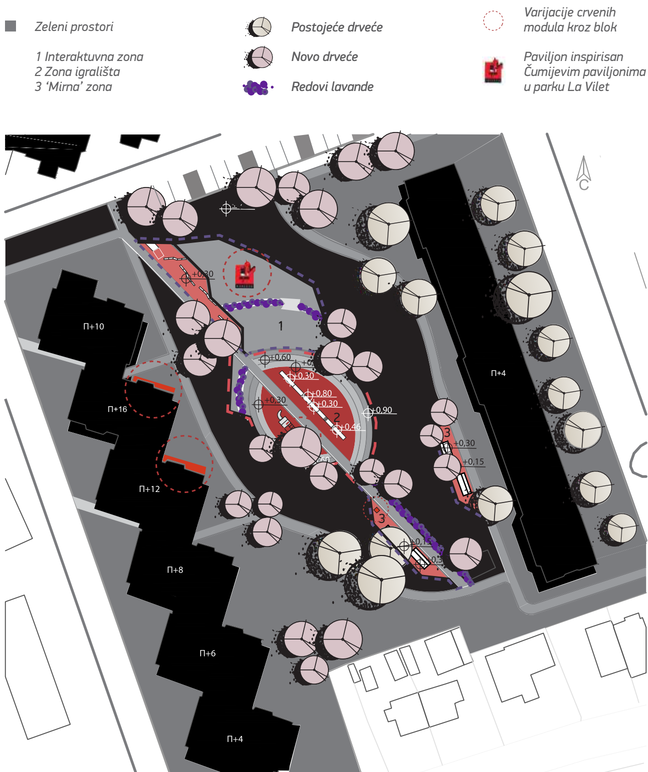
Slika 63. Situaciono rješenje prostornog obuhvata dijela otvorenih prostora stambenog naselja Borik, Banja Luka, studentski rad Anastasije i Teodore Vuletić, studijski program Arhitektura, školska godina 2024-2025, Arhitektonsko-građevinsko-geodetski fakultet, Univerzitet u Banjoj Luci
